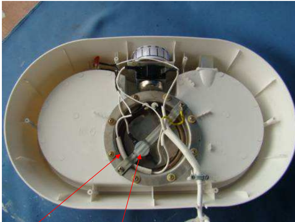
Thermal link
