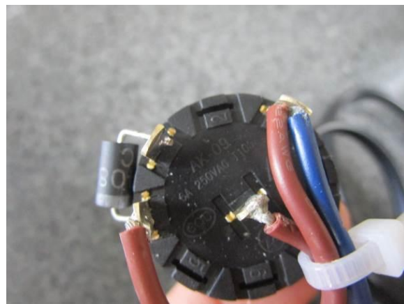
61). Speed switch
