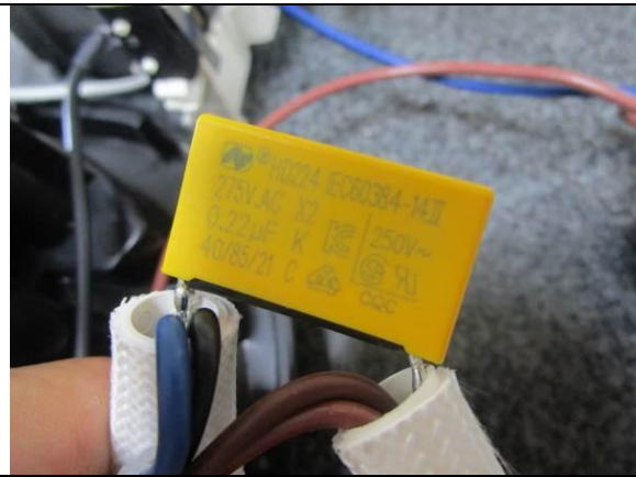
63). X capacitor
