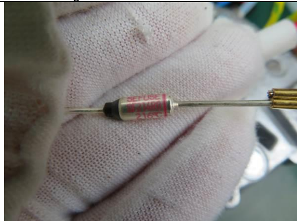
195. Thermal link
