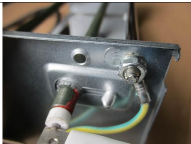
44). Earthed marking
