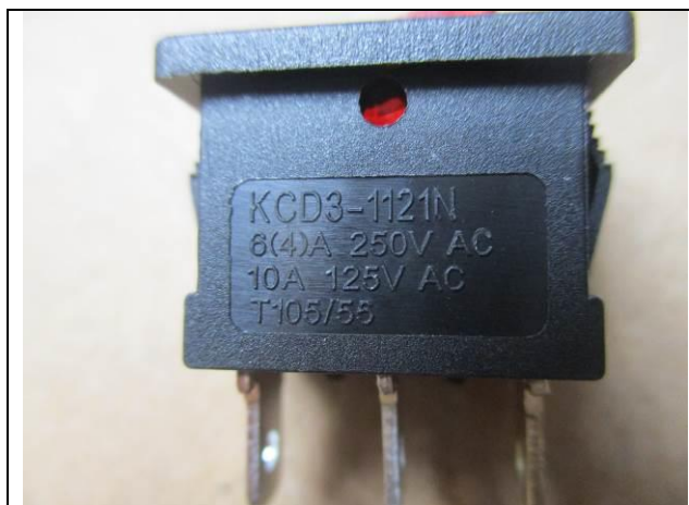
49). Switch
